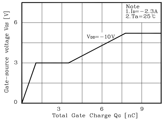
Fig. 6 V_{GS} - Q_G
